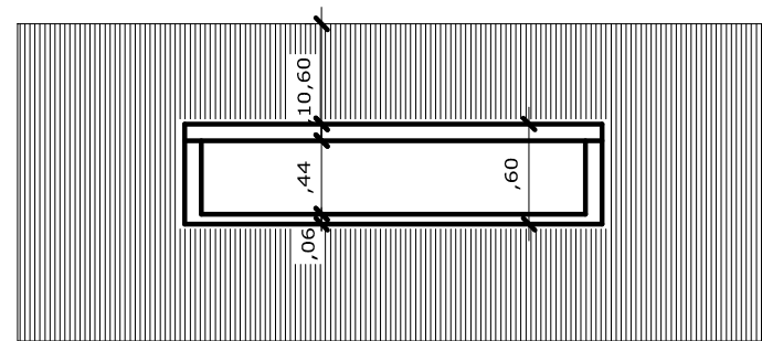
3 CORTE CARNEIRA ADULTO 1:50
